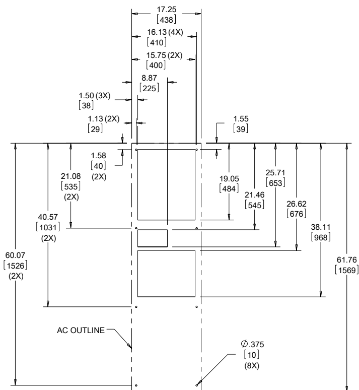
Cutout Dimensions
