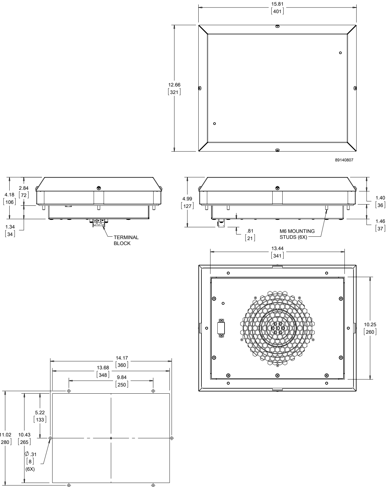
Cutout Dimensions
