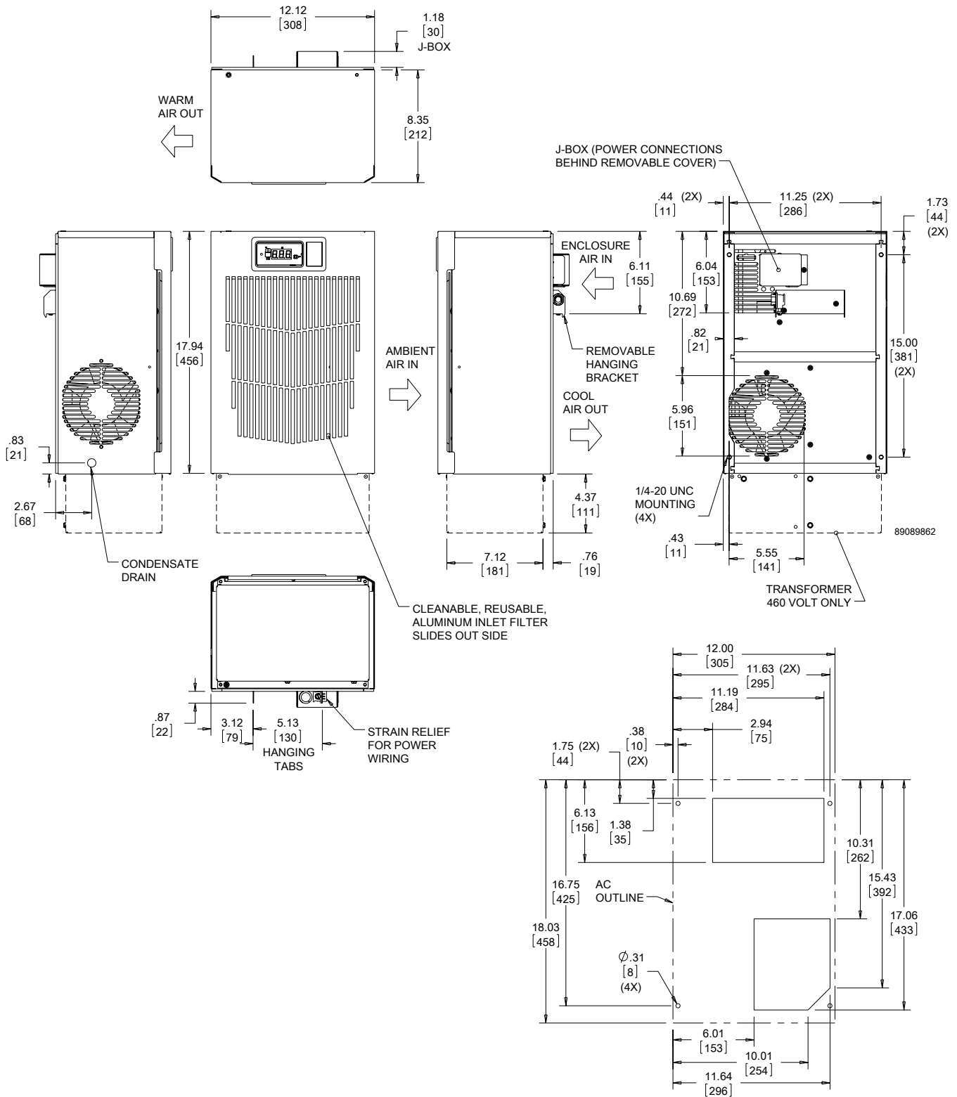
Cutout Dimensions
