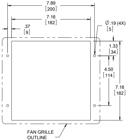
CUTOUT DIMENSIONS
