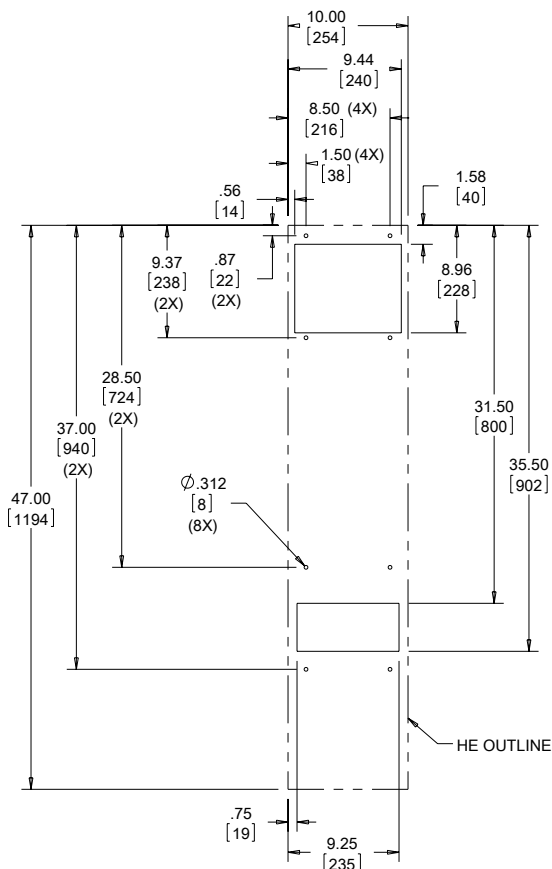
Cutout Dimensions
