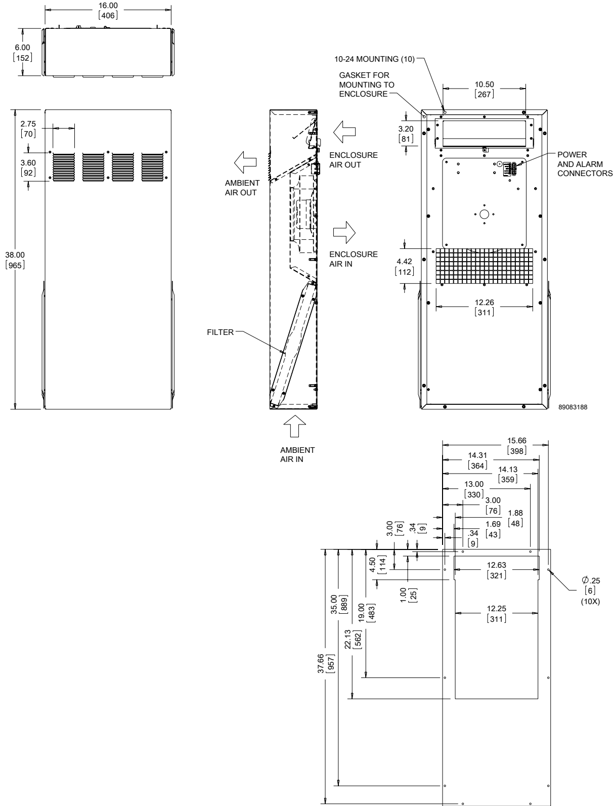
CUTOUT DIMENSIONS
