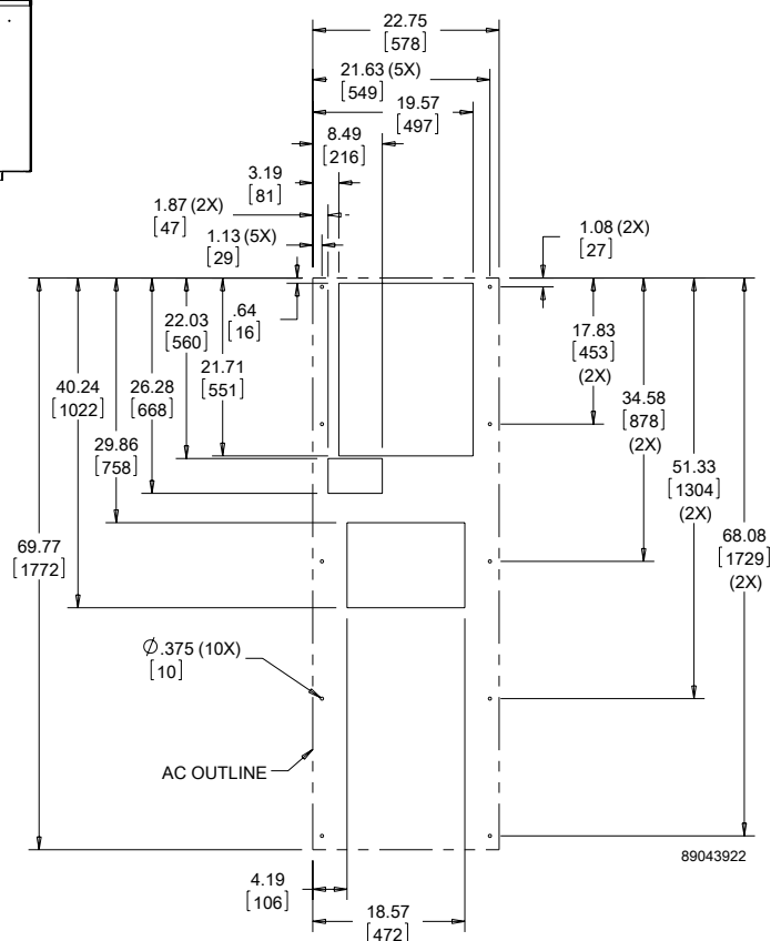
Cutout Dimensions
