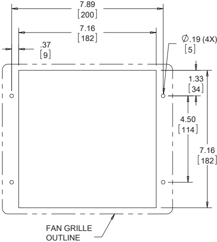
CUTOUT DIMENSIONS
