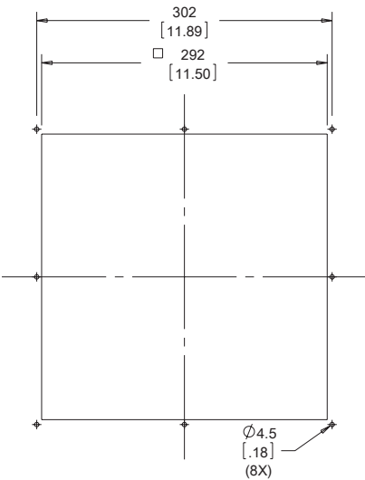
CUTOUT DIMENSIONS
