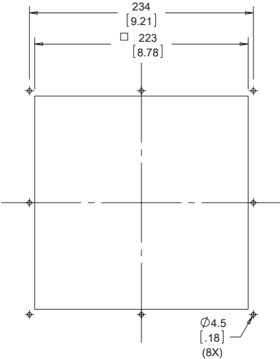
CUTOUT DIMENSIONS
