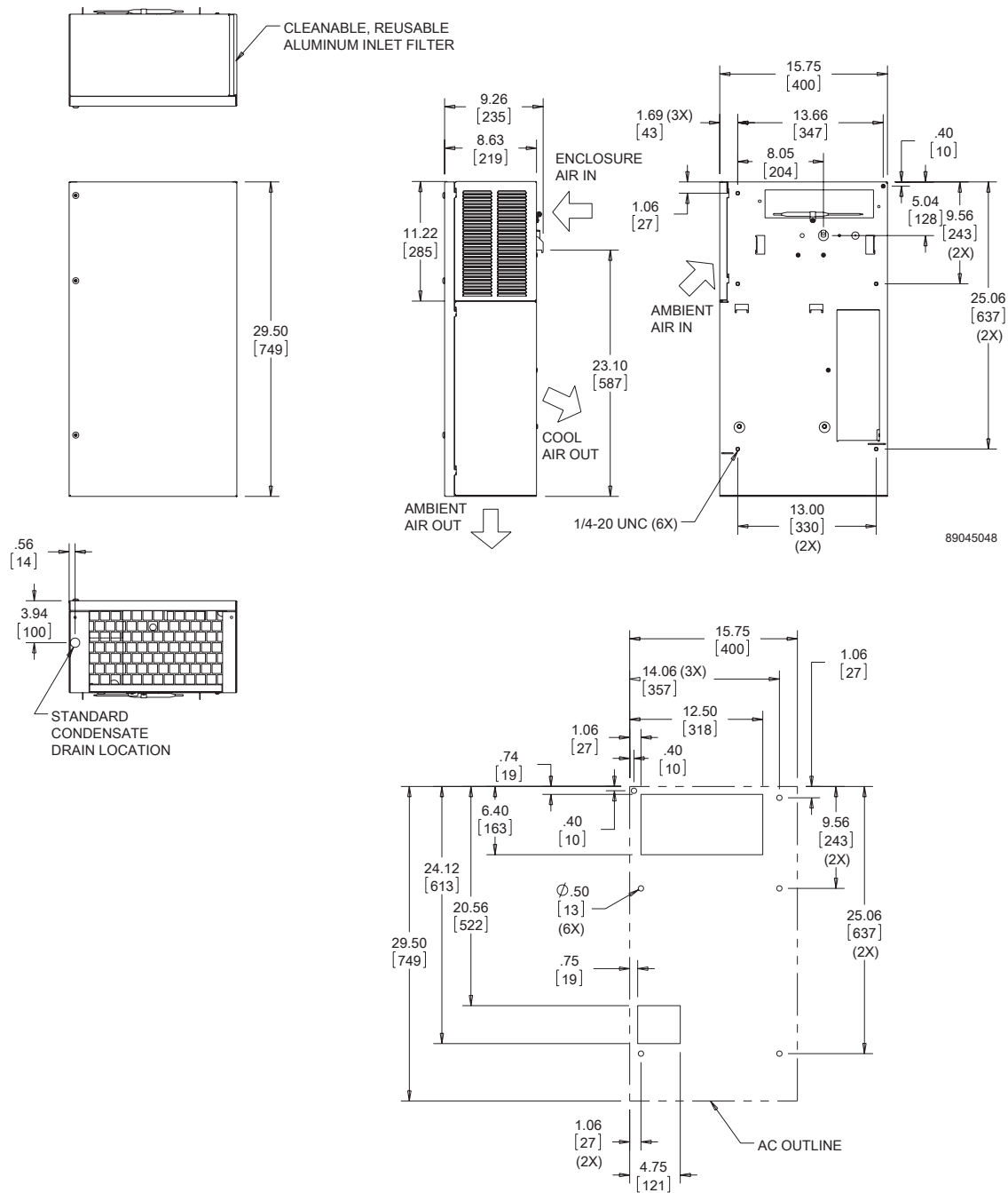
Cutout Dimensions
