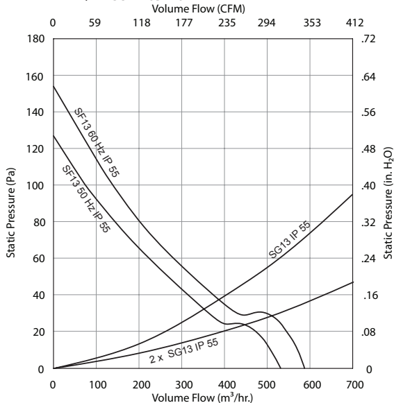
TYPE 12 / IP 55 Filter Fan
