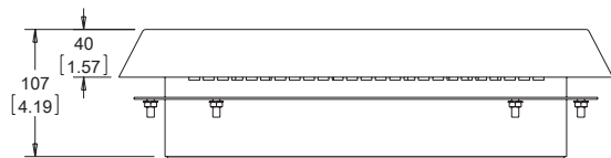
Filter Fan SR16 28 CFM (475 m 3 /hr.)
