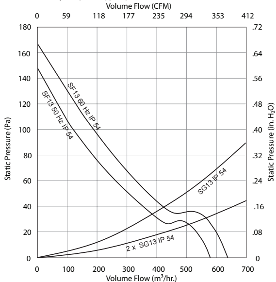
TYPE 12 / IP 54 Filter Fan
