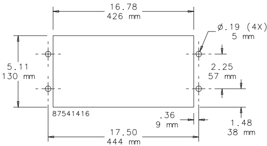
CUTOUT DIMENSIONS
