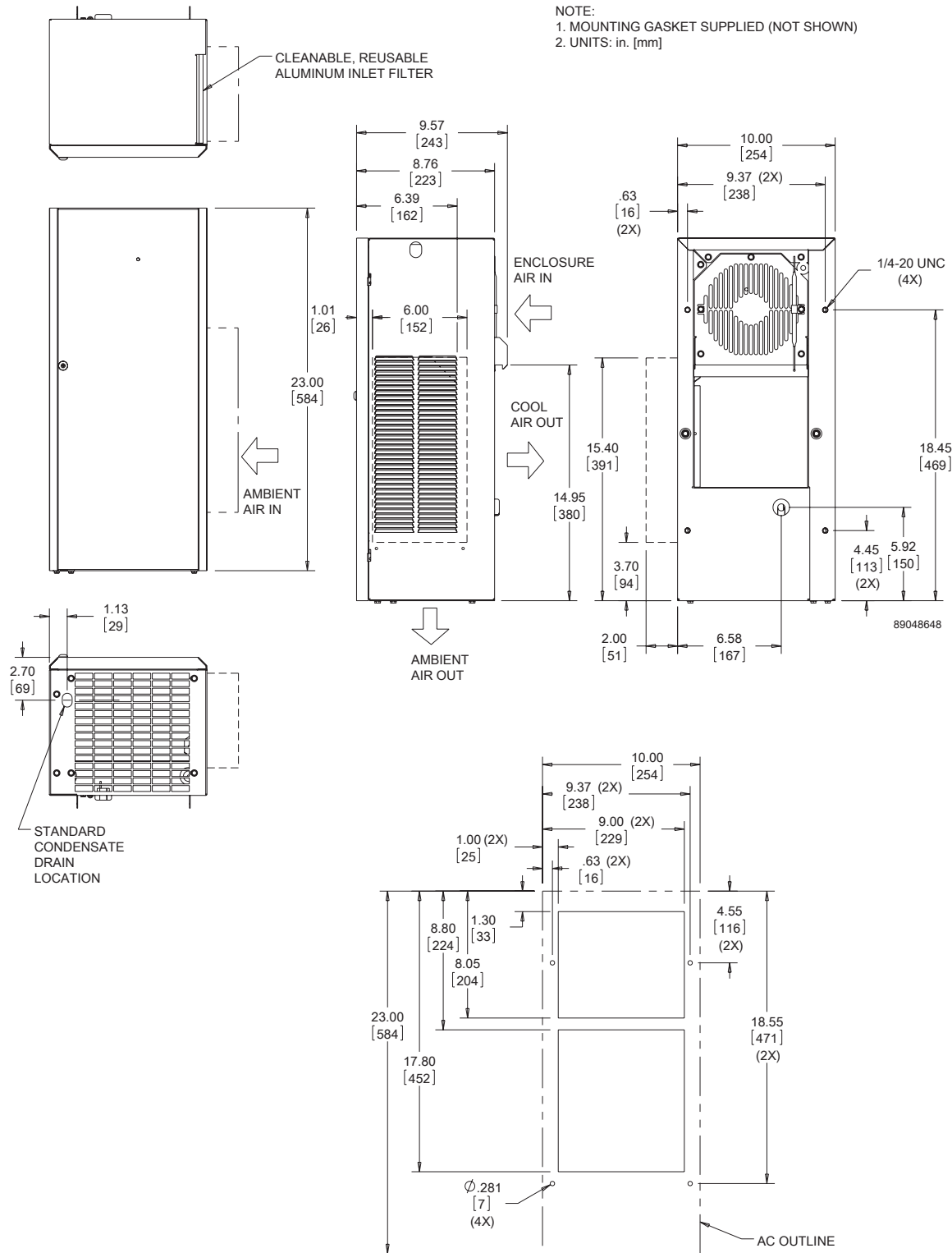
Cutout Dimensions
