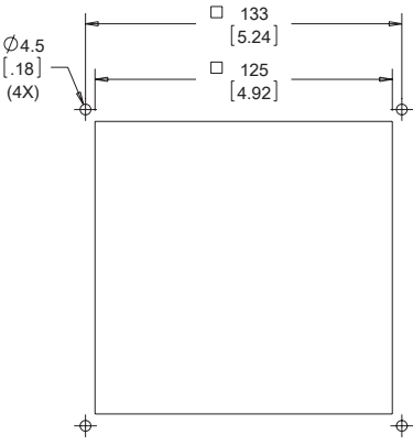
CUTOUT
