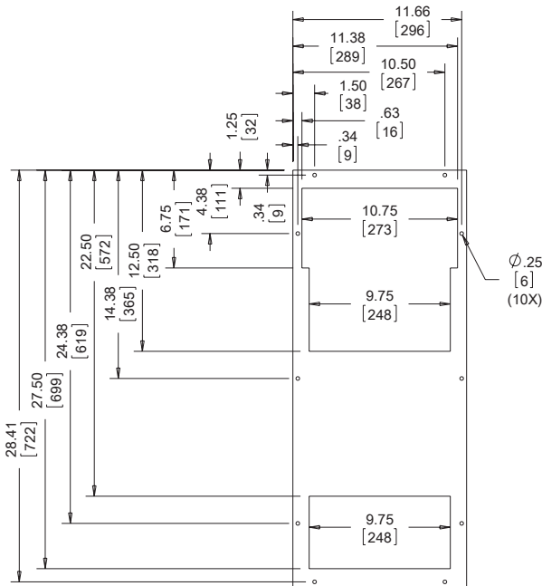
CUTOUT DIMENSIONS
