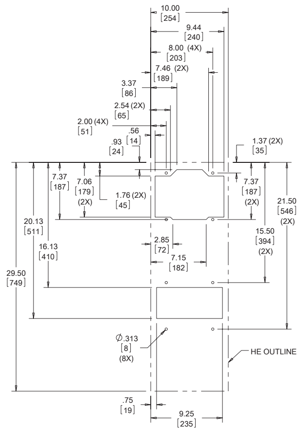
Cutout Dimensions
