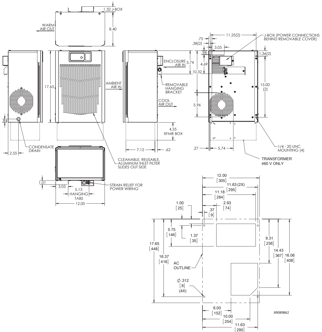
Cutout Dimensions
