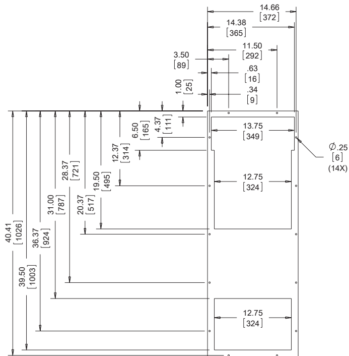
CUTOUT DIMENSIONS
