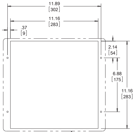
FAN GRILLE OUTLINE
