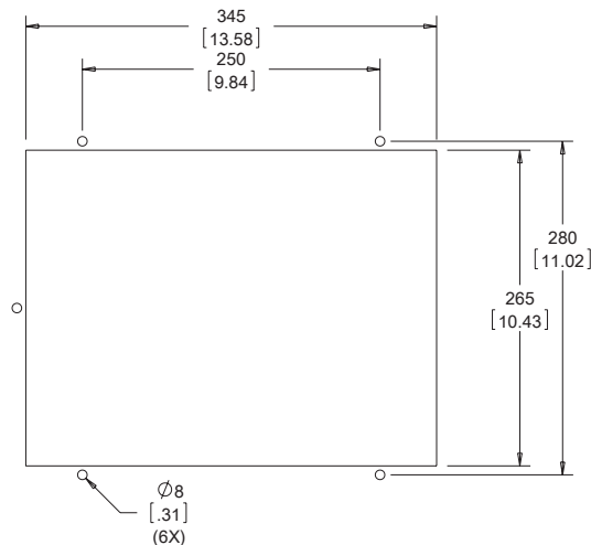
CUTOUT DIMENSIONS
