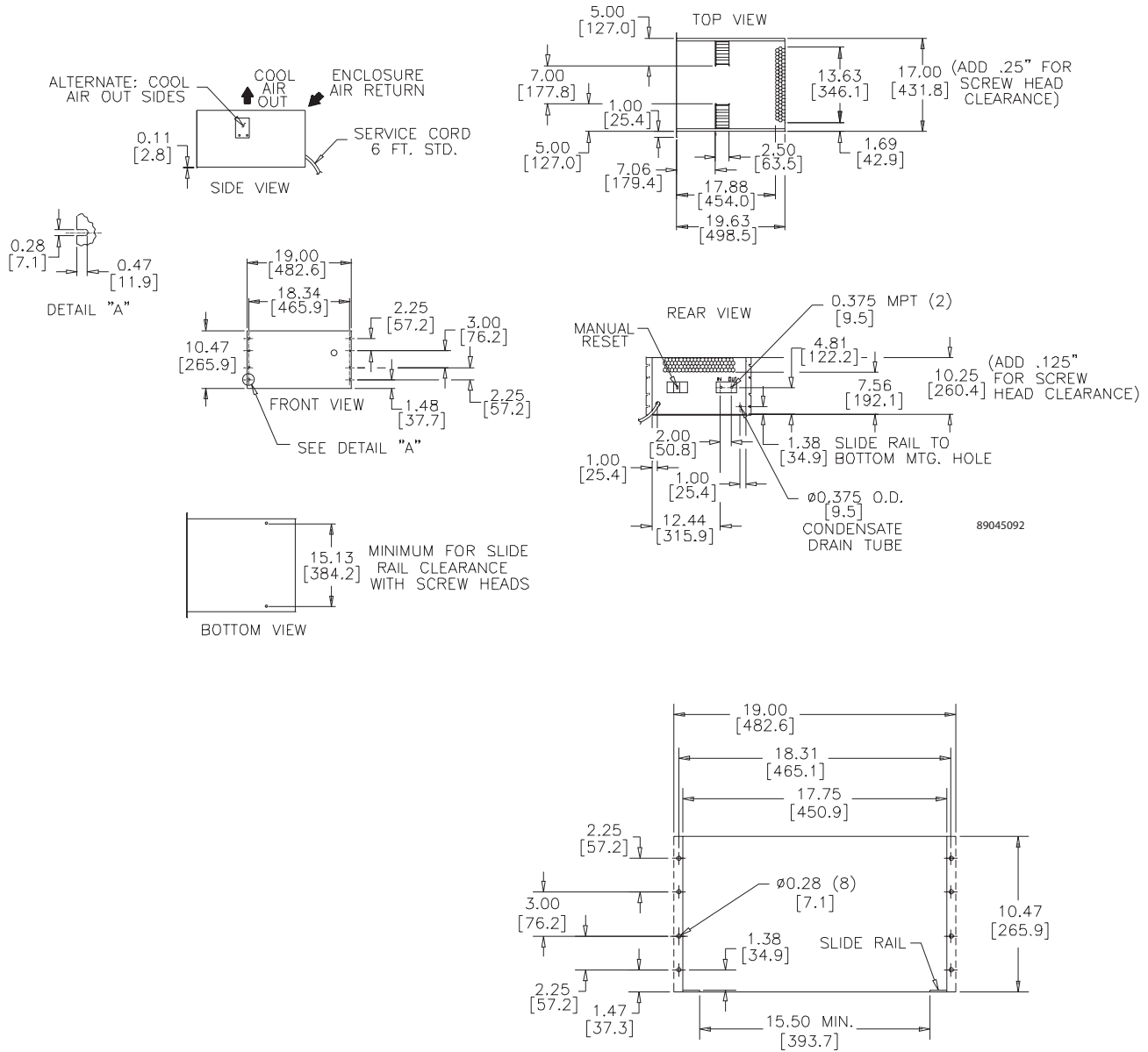
Cutout Dimensions
