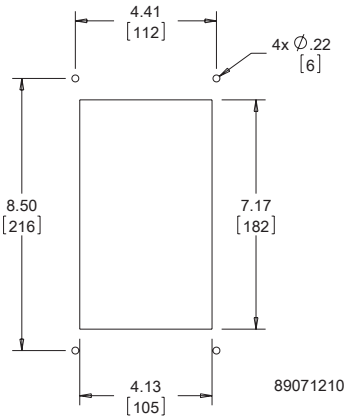
Cutout Dimensions
