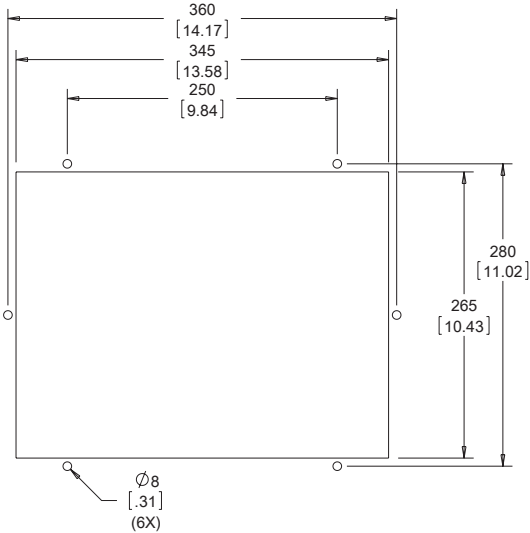
CUTOUT DIMENSIONS
